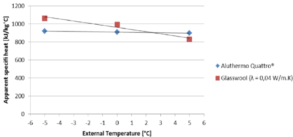
Figure 13 – évolution de la chaleur spécifique par rapport à la température extérieure pour Aluthermo Quattro® et la laine de verre λ0,04
