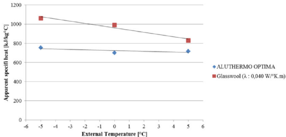
Afbeelding 13 – de evolutie van de specifieke schijnbare warmte in vergelijking met de buitentemperaturen voor Aluthermo Optima® en glaswol \lambda 0,04
